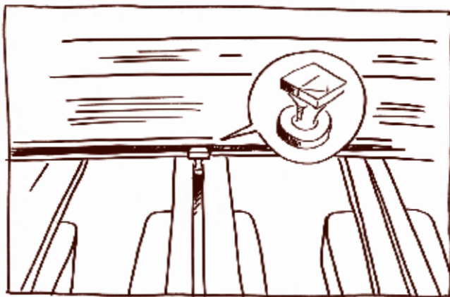
Schritt 3: Biowert Clip. Er verbindet die Terrassendielen mit den Grundprofilen.
